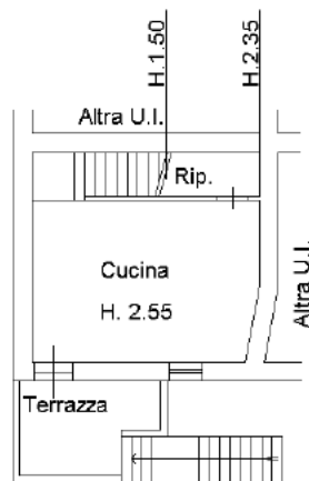
PIANTA PIANO PRIMO
