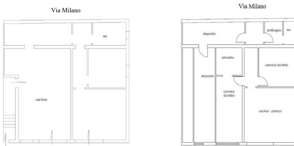
Fig. 25- Piano terra sub 3 (il piano risulta seminterrato) - Confronto tra la planimetria catastale e stato di fatto.
