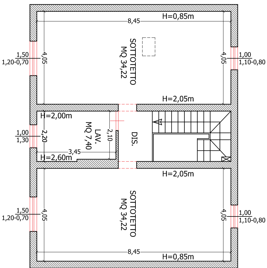
PIANO SECONDO (SOTTOTETTO)
