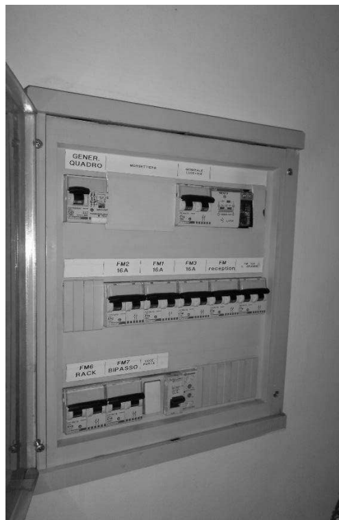
FOTO n°16 – QUADRO ELETTRICO ALL'INGRESSO
