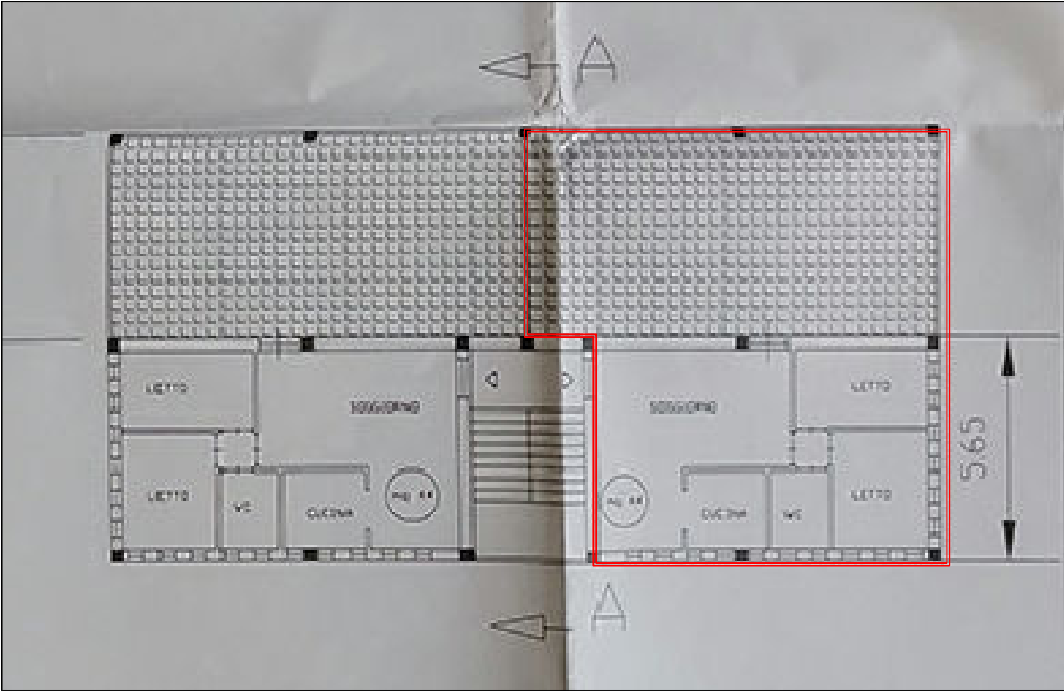
PIANTA PIANO TERZO SOTTOTETTO
