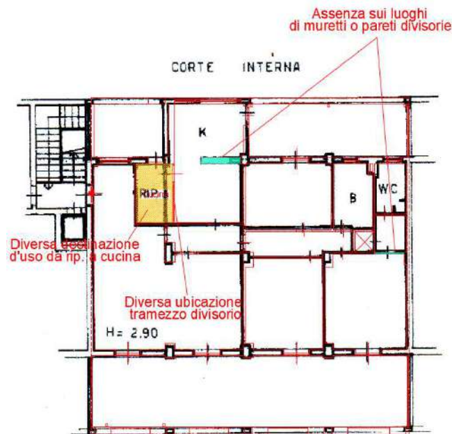
Fig. 8- Sovrapposizione della planimetria di rilievo con la planimetria catastale
