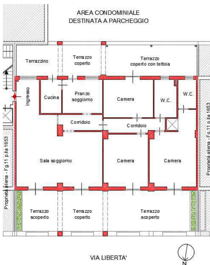
Fig.4 – Planimetria dello stato attuale
