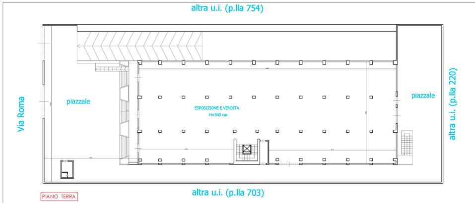
Capannone oggetto di pignoramento: Rilievo dello stato dei luoghi – PIANO TERRA
