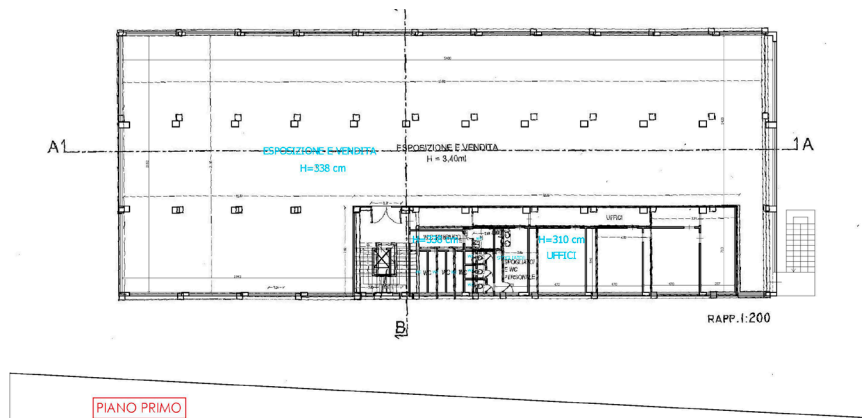
Sovrapposizione planimetria di progetto di SCIA e rilievo dello stato dei luoghi – PIANO PRIMO
