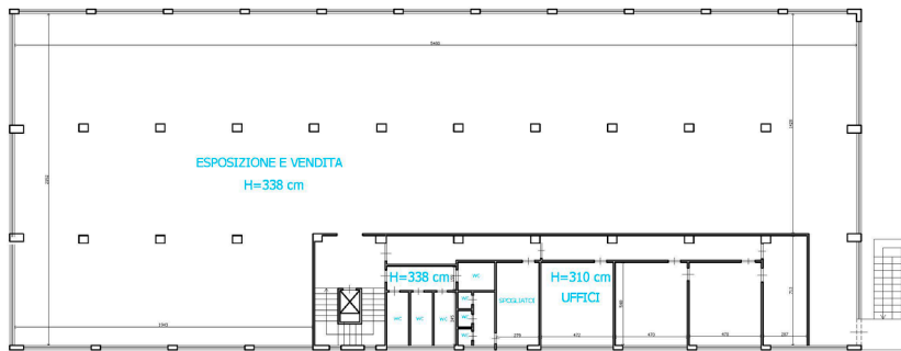
Capannone oggetto di pignoramento: Rilievo dello stato dei luoghi – PIANO PRIMO
