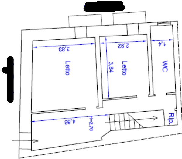
Comune di Vizzini foglio 80 part. PIANO TERRA
