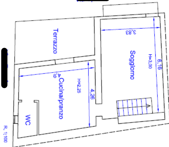
PIANO PRIMO
