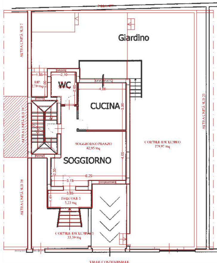
PIANTA PIANO TERRA H=2,70m
