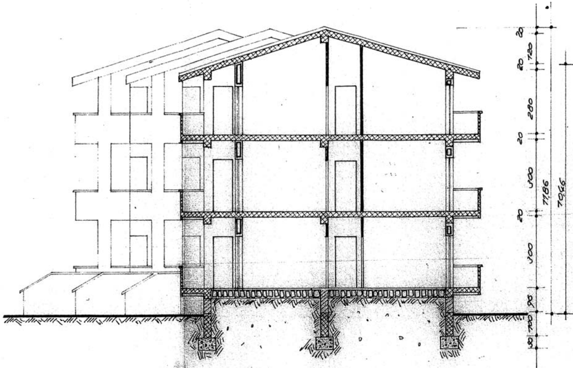
SEZIONE A-A
