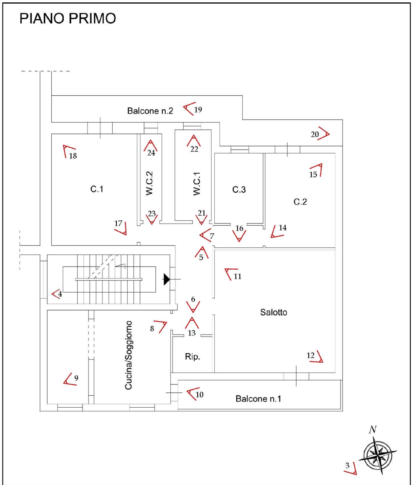
Figura 2: Coni ottici delle foto a seguire (U.I. al piano primo)
