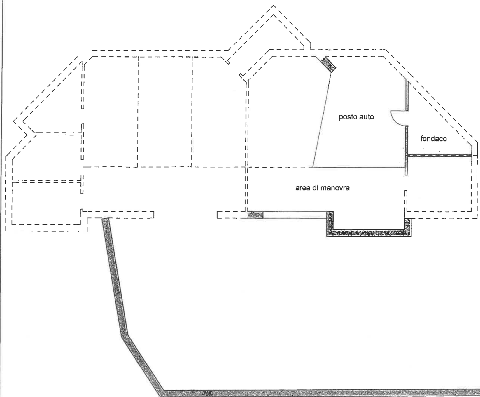
Piano Interrato Scala 1:100
