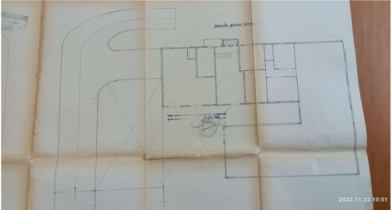
Pianta del piano terra
