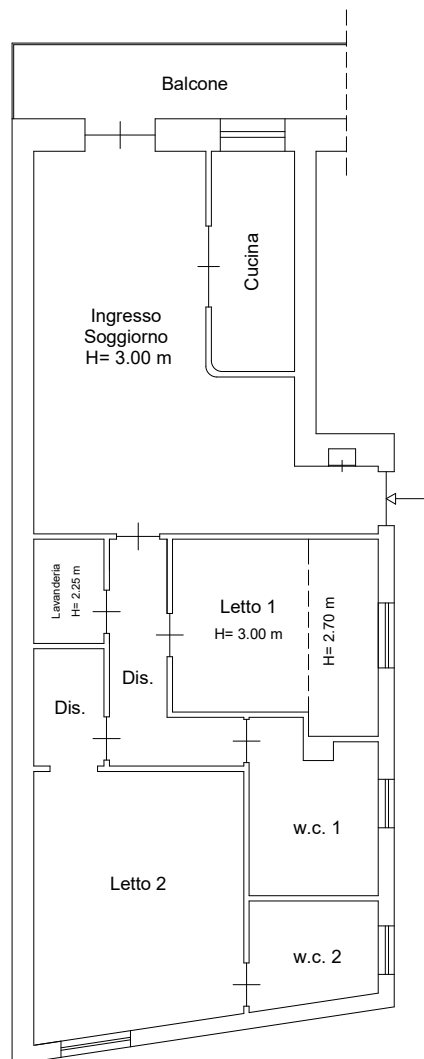
PLANIMETRIA APPARTAMENTO
