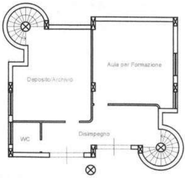
Fig. 2 - Planimetria Piano Seminterrato
