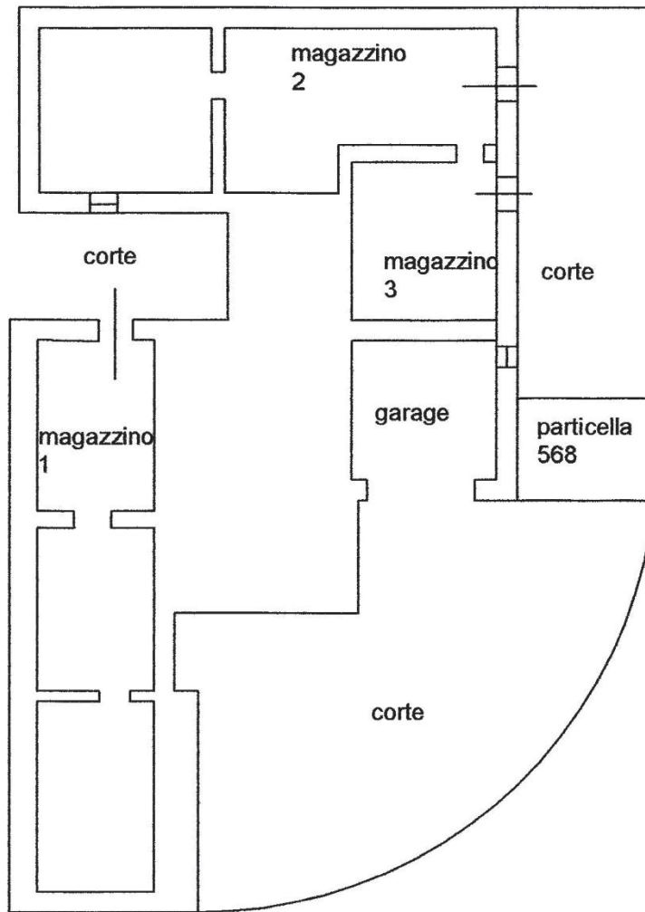
pianta piano seminterrato
