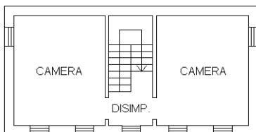
PIANO SECONDO (P2) - H=236
