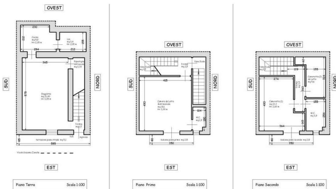
Figura 8 – Stralcio piante di rilievo (Immobile piano terra, primo e secondo Fig. 69, part. 13233, sub. 1)
