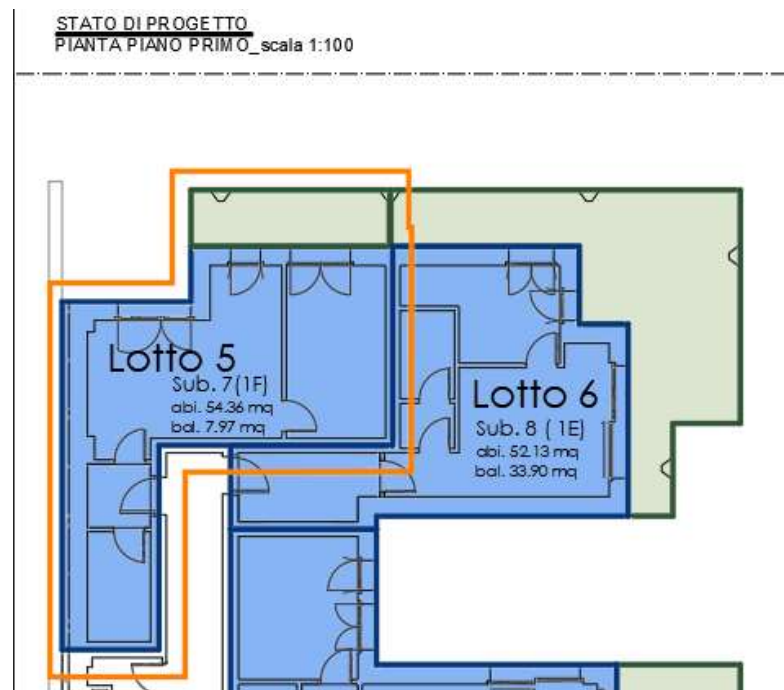
Stralcio planimetria abitazione Sub. 7 – piano primo
