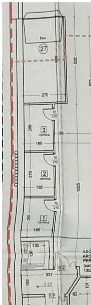
PdC n.245 del 2018 piano primo interrato
