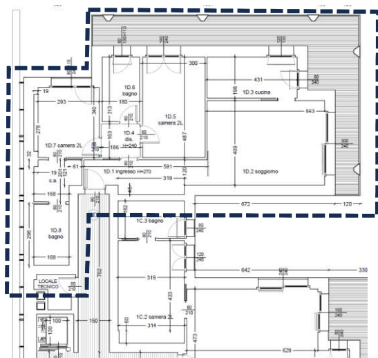
Stralcio planimetria piano primo SCIA 2019 stato autorizzato con PdC 2018
