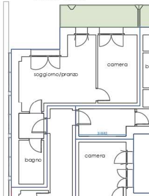
Planimetria dell'abitazione sub. 7 – piano primo
