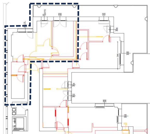
Stralcio planimetria piano primo SCIA 2019 stato sovrapposto
