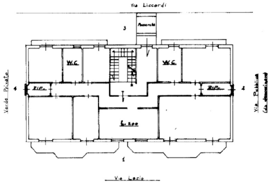
PIANTA 1° PIANO
