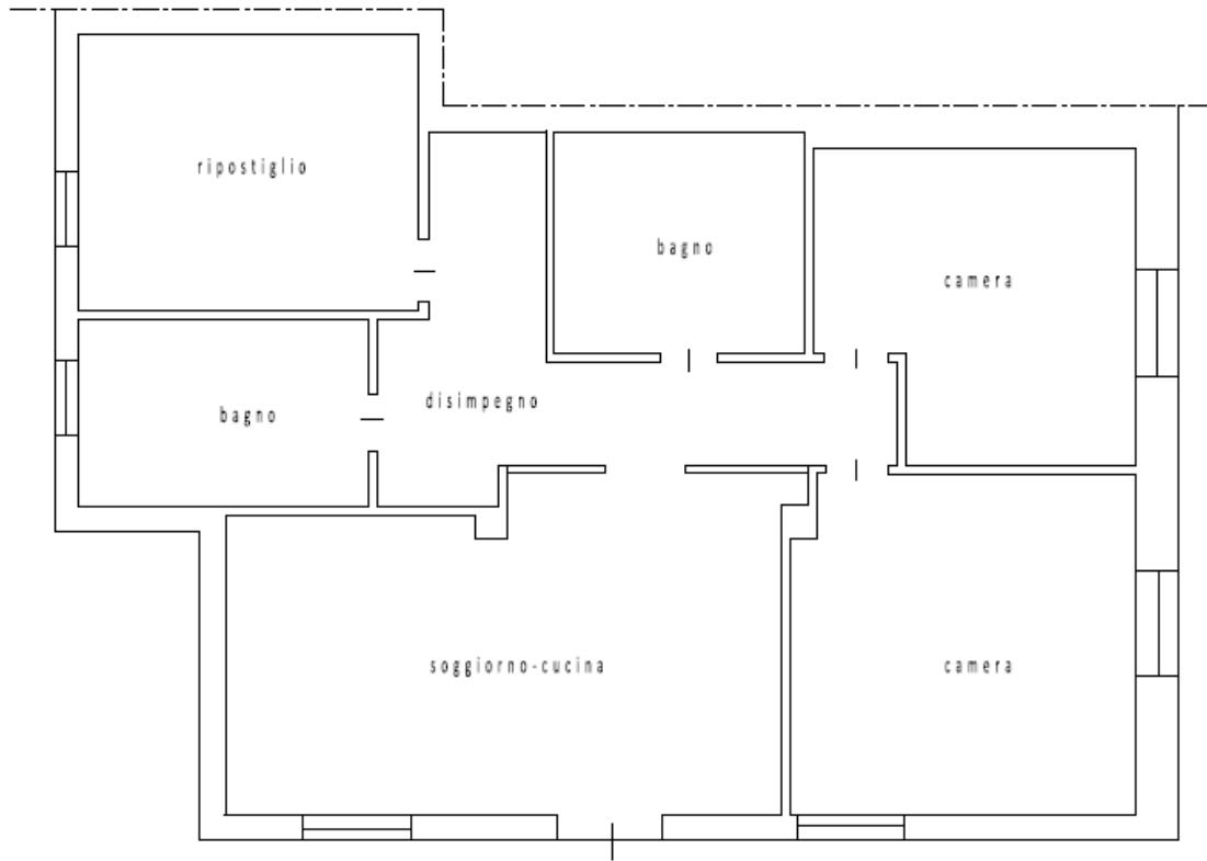
PIANTA PIANO TERRA-SOTTOSTRADA STATO DI FATTO
