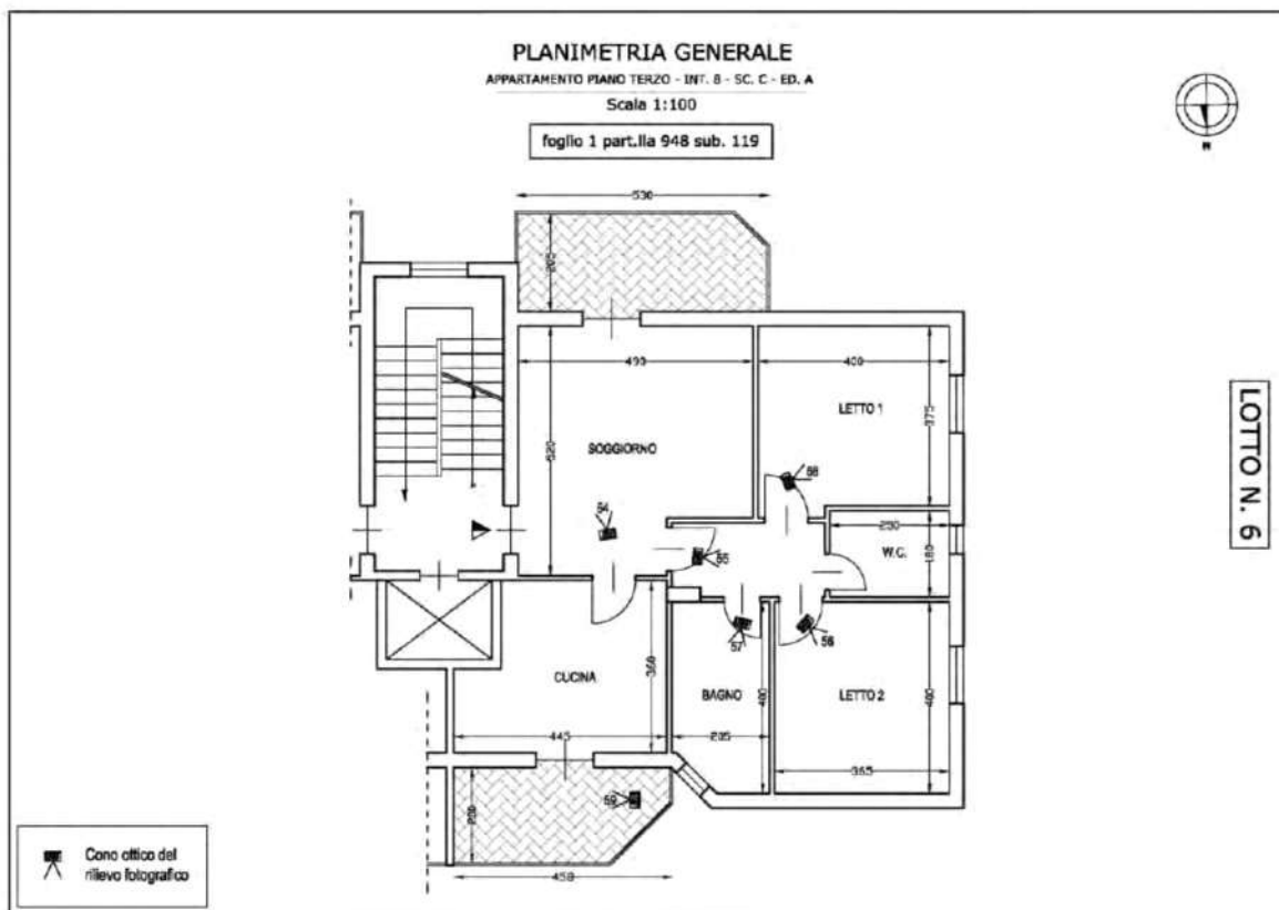
Figura 1 – Planimetria appartamento
