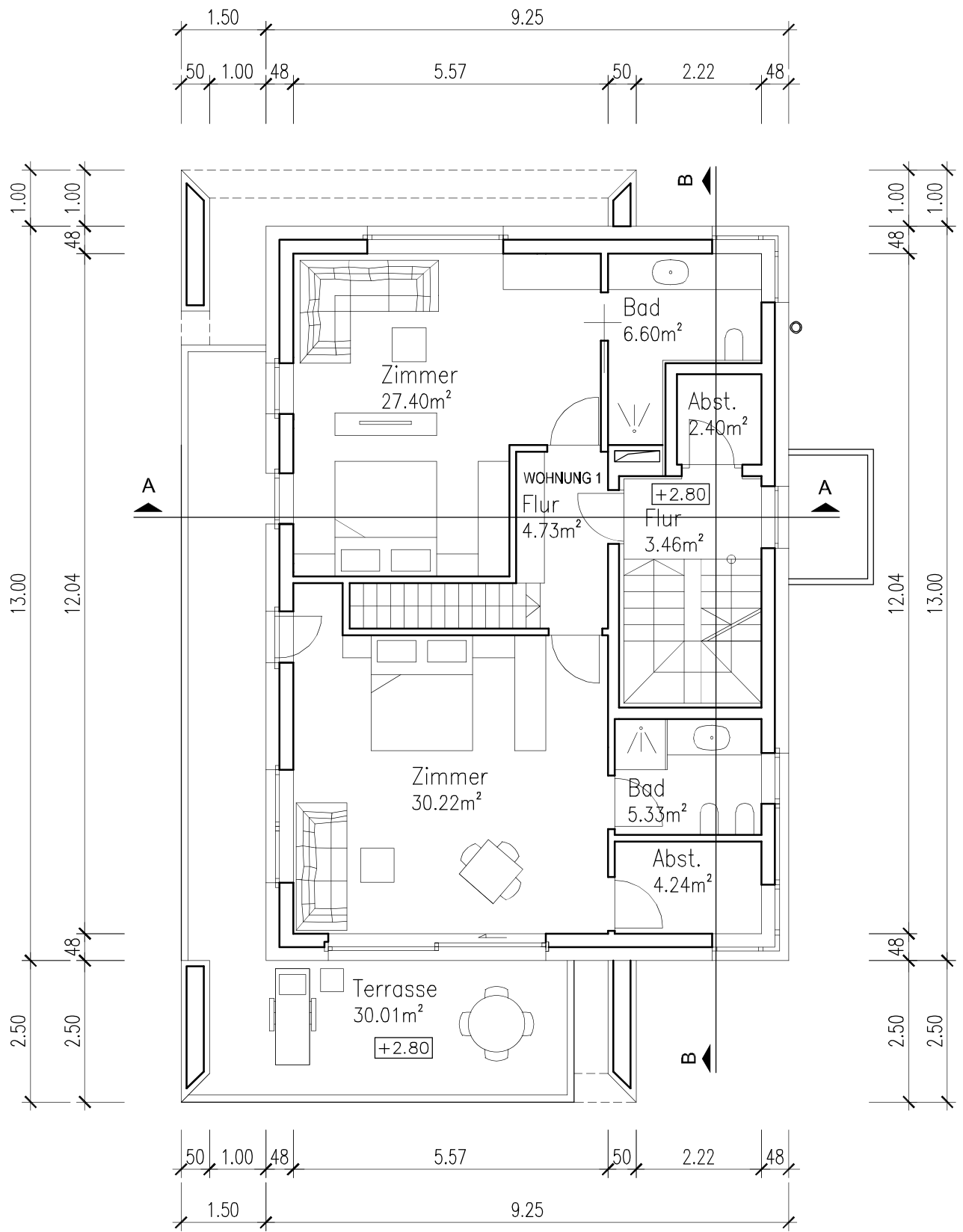
OBERGESCHOSS 1:100
