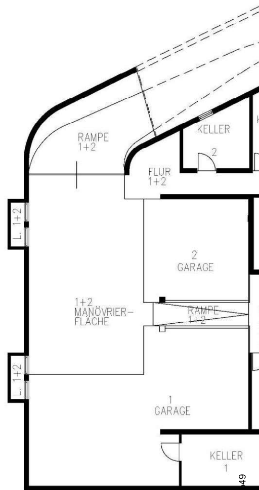
KELLERGESCHOSS - PIANO INTERMEDIO
