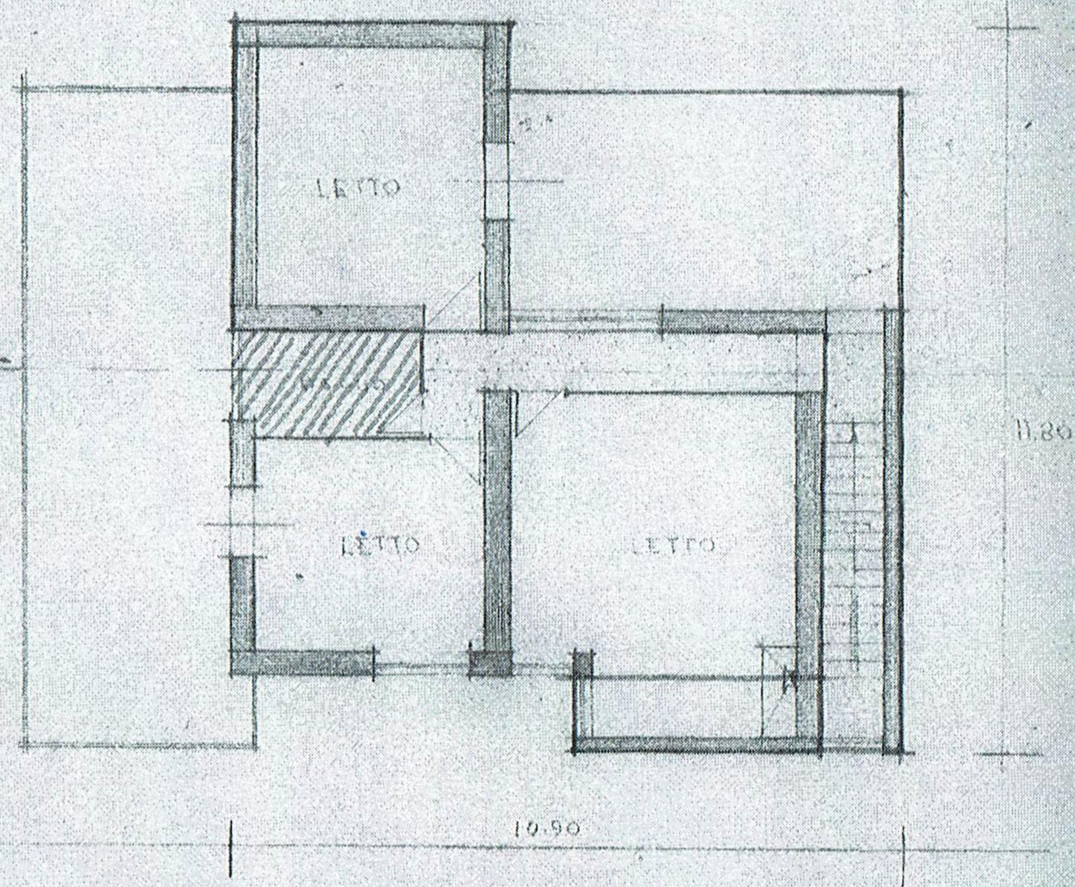
Pianta Secondo Piano
