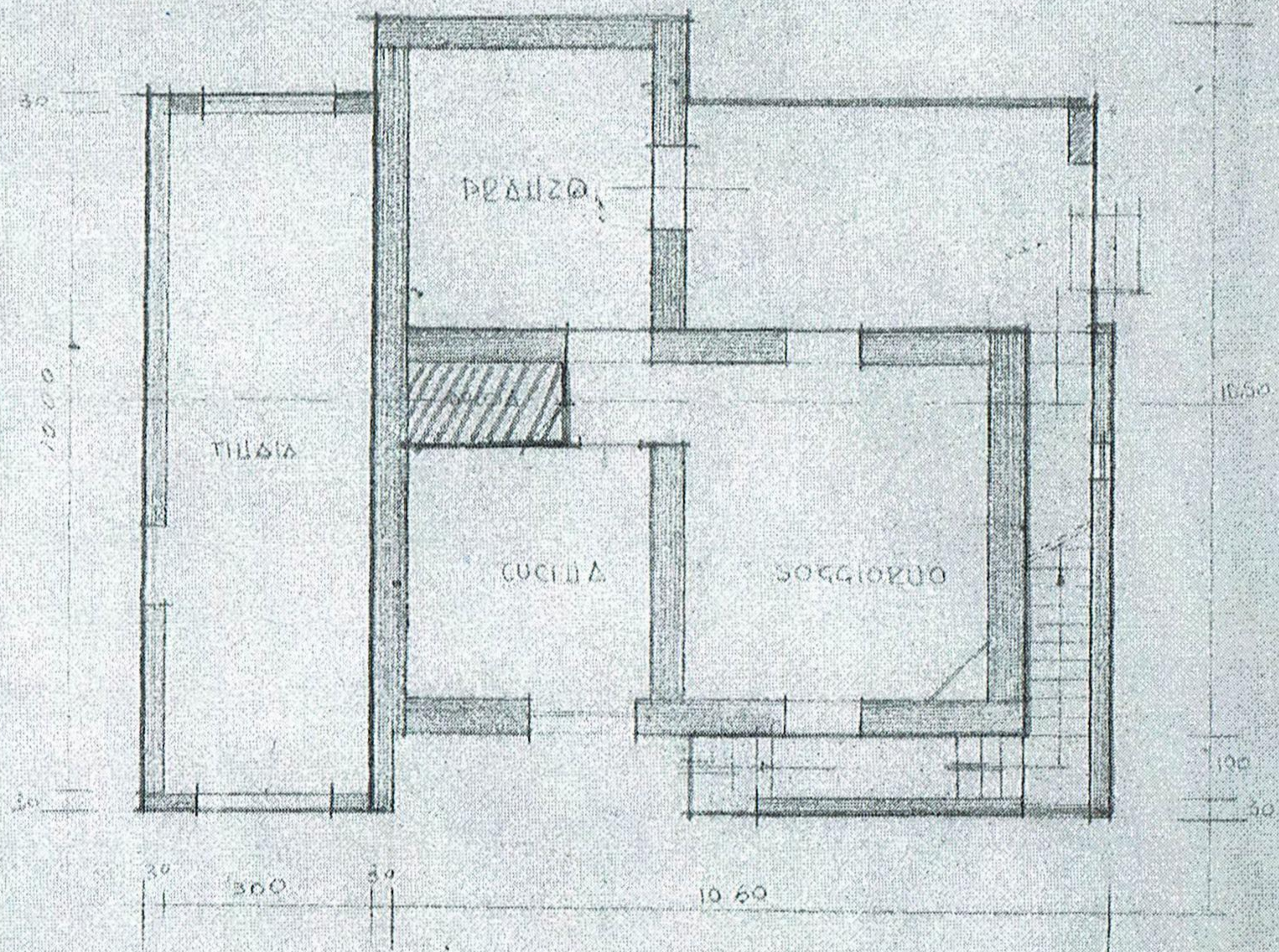
Pianta Primo Piano
