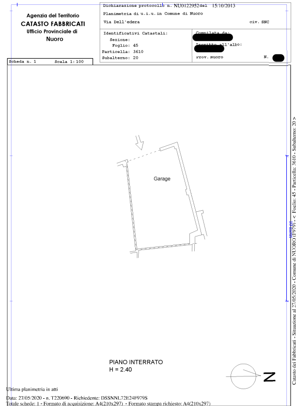
F-01 Subalterno 20 1:100
