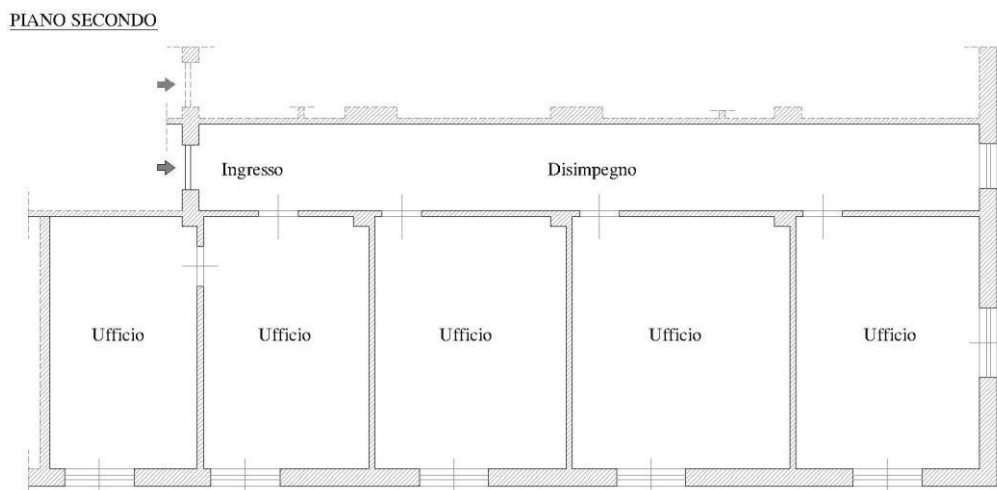
Fig. 9 – Planimetria Uffici piano secondo
