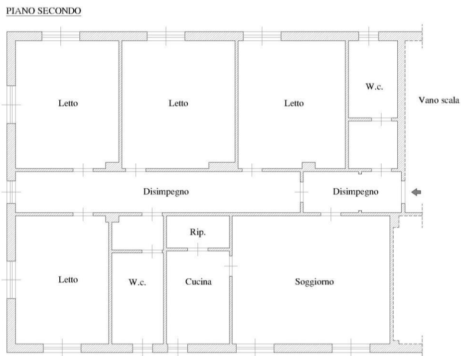
Fig. 7 – Planimetria Abitazione (n.1) piano secondo
