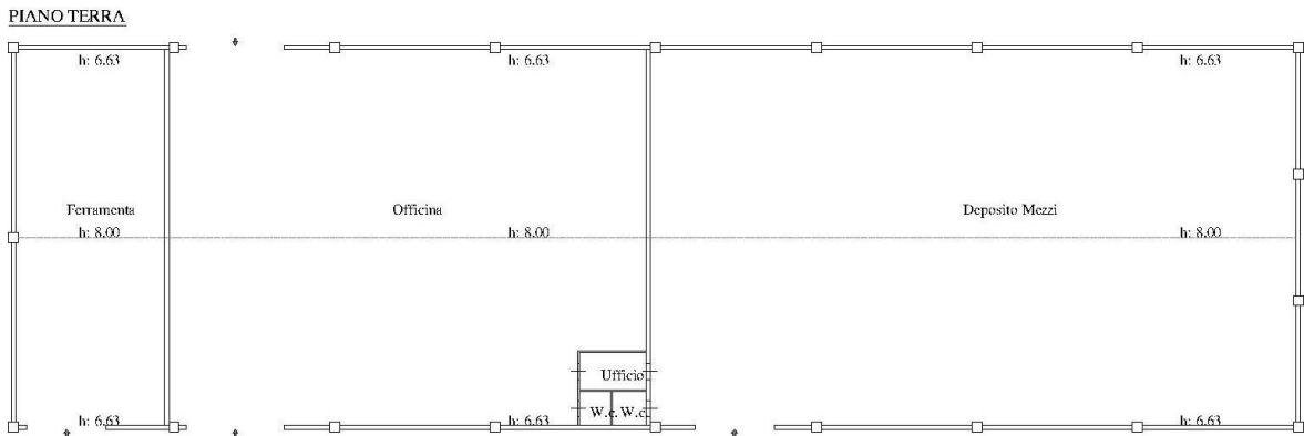
Fig. 11 – Planimetria capannone (n.2) piano terra
