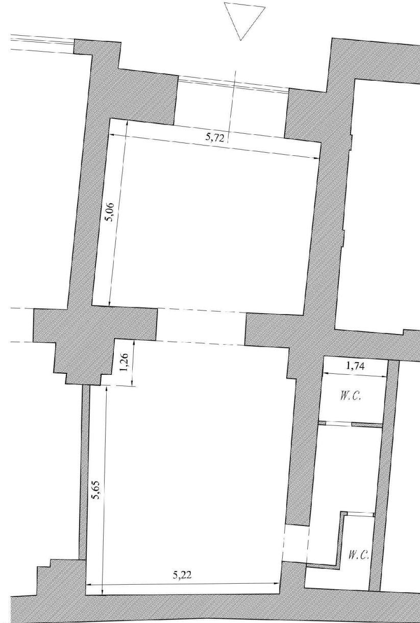
Rilievo metrico Negozio
