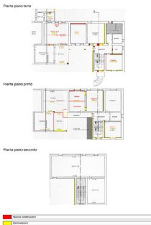
Schema di massima con individuazione delle difformità edilizie
