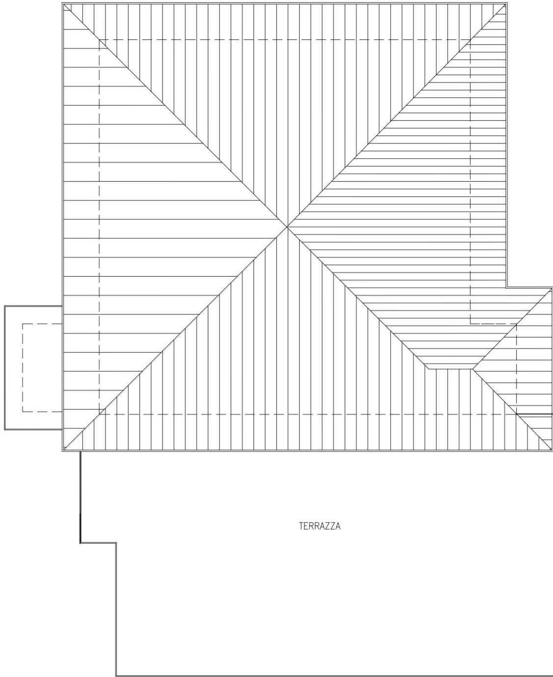
PIANTA COPERTURA Rilievo indicativo e non esaustivo
