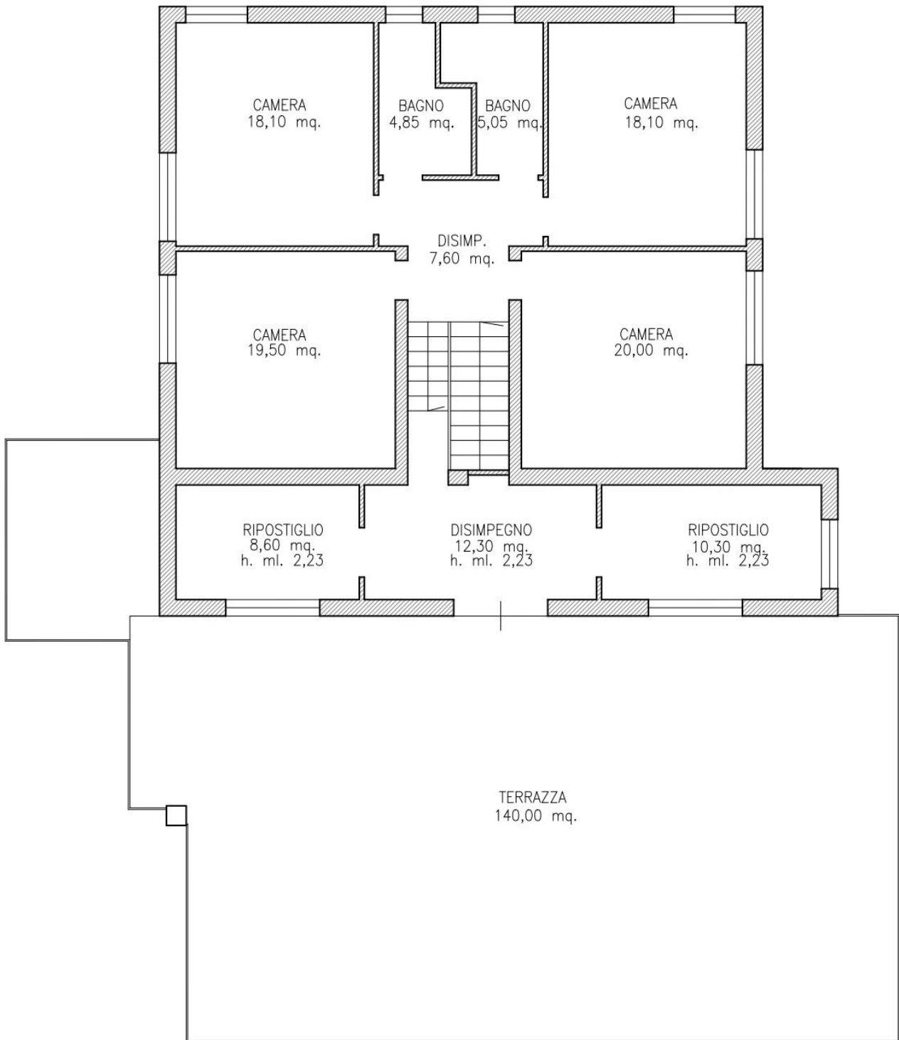
PIANO PRIMO Rilievo indicativo e non esaustivo H. ml. 3,00
