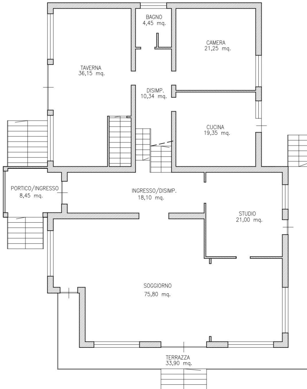
PIANO TERRA-RIALZATO Rilievo indicativo e non esaustivo H. ml. 3,00
