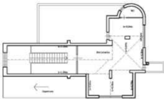
PIANO SECONDO/SOTTOTETTO rilievo
