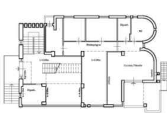
PIANO TERRA-rilievo
