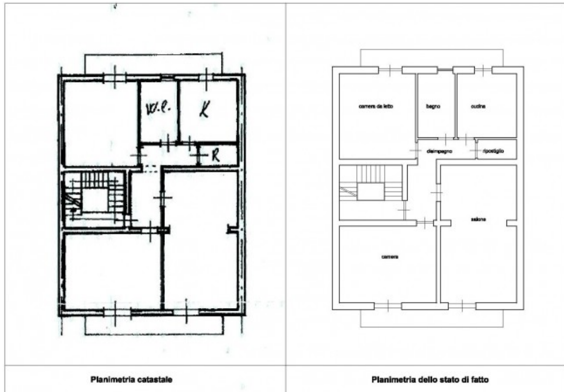
CONFRONTO PLANIMETRIA CATASTALE-PANIMETRIA DELLO STATO DI FATTO
