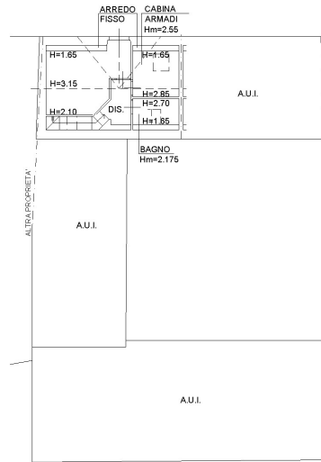
PIANTA PIANO SECONDO
