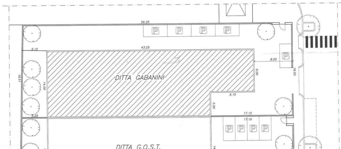
PLANIMETRIA VERDE E PARCHEGGI SCALA 1:200
