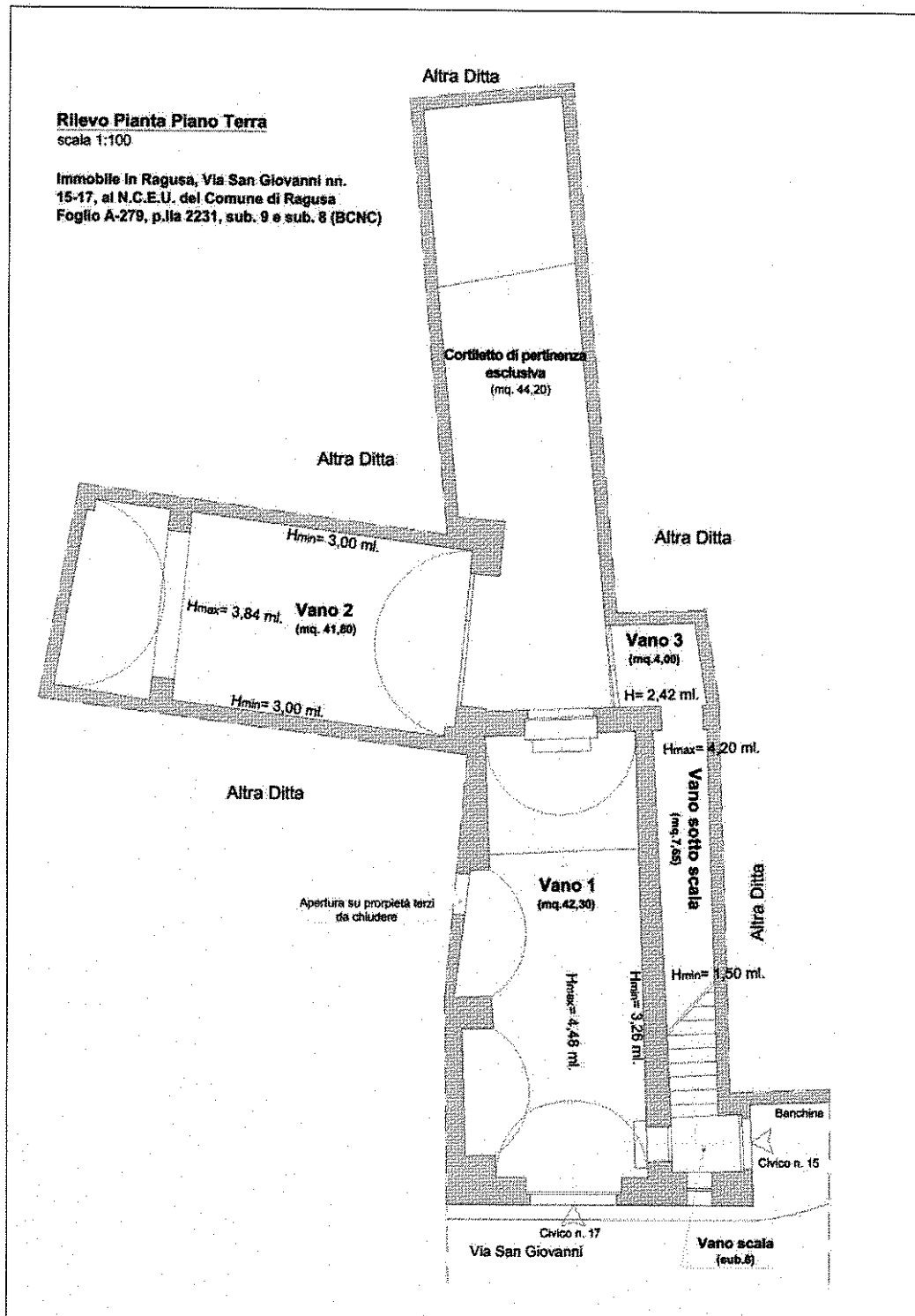
Rilevo Pianta Piano Terra
