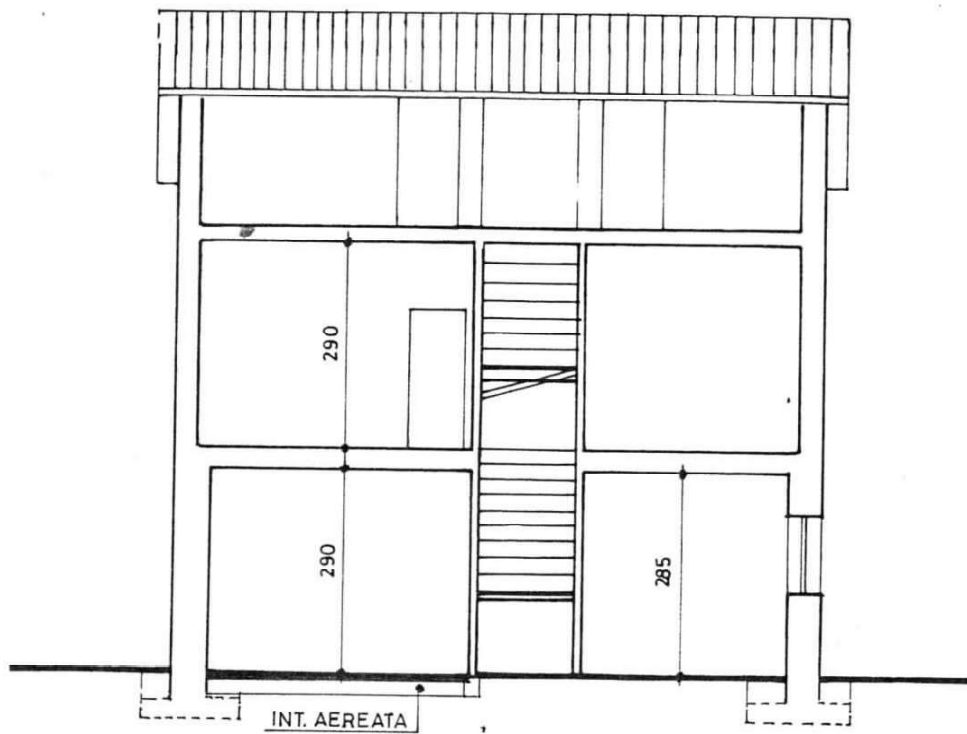
SEZIONE A-A
