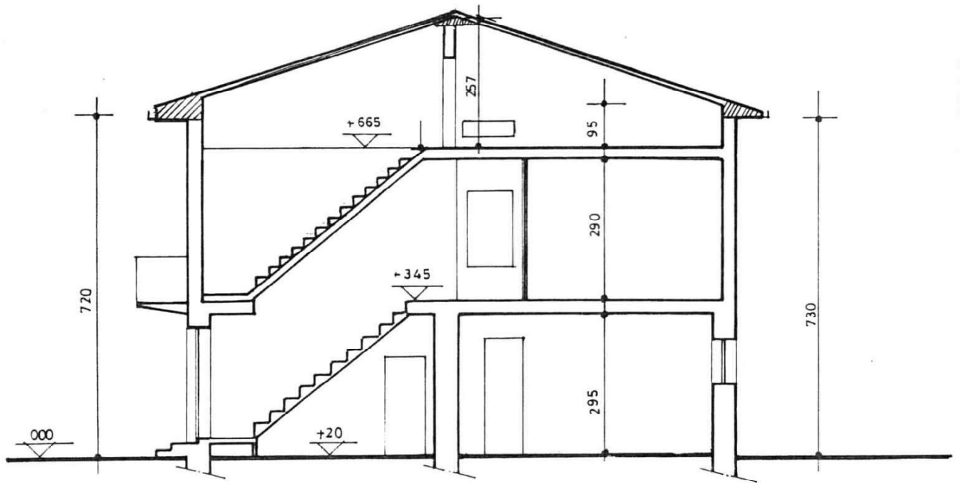
SEZIONE B-B
