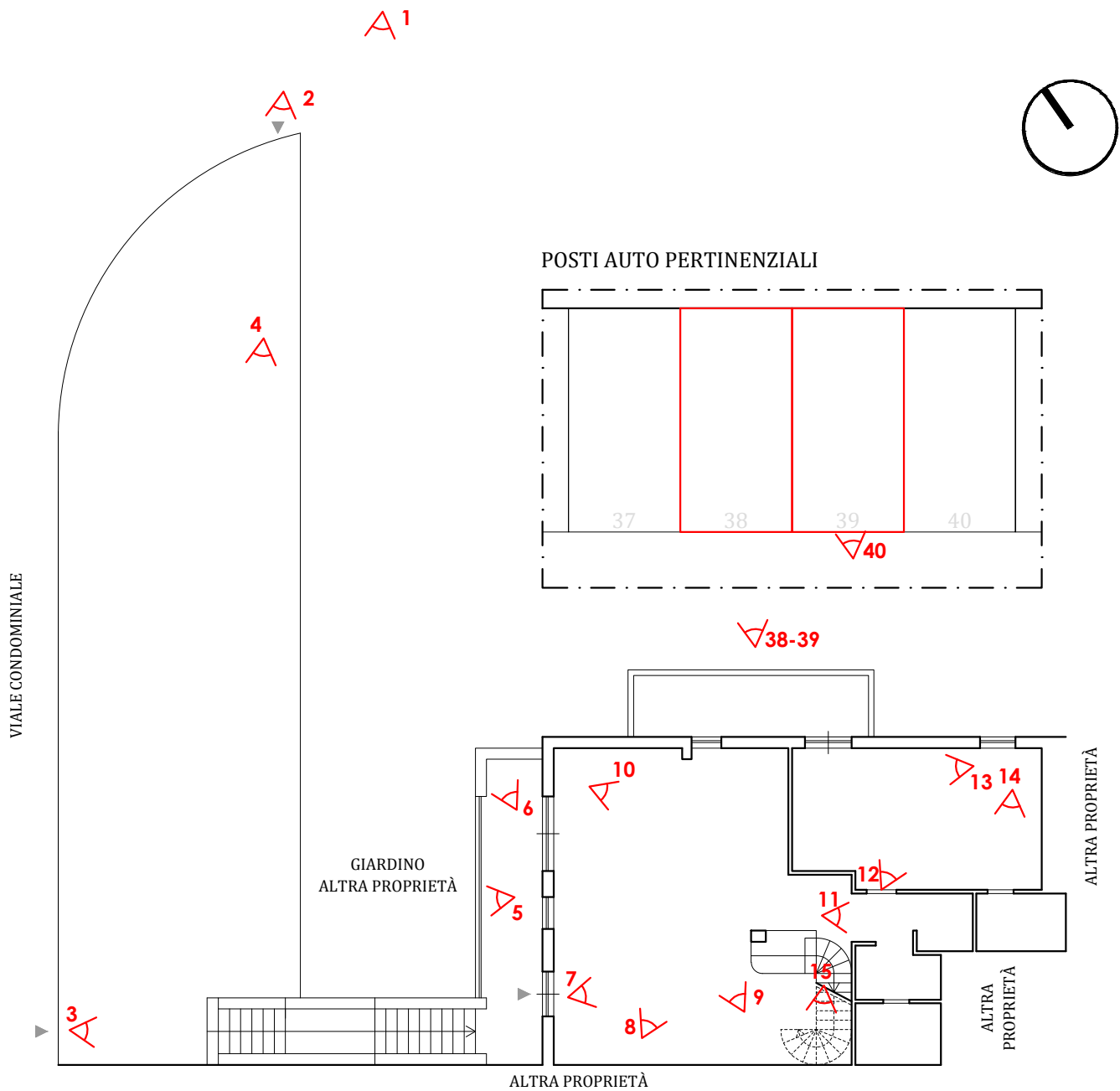
PIANTA PIANO TERRA_interpiano h. 3,00 m
