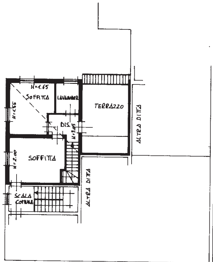
PIANO SOTTOTETTO
