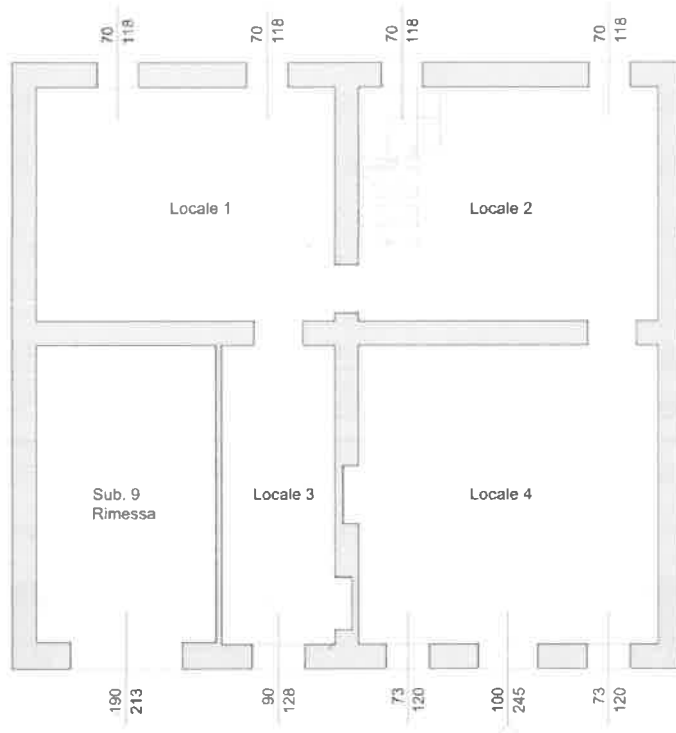
Fot. 1 - Pianta piano terra
