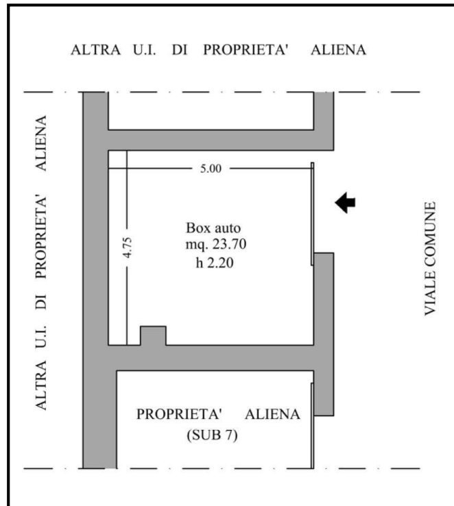
RILIEVO METRICO
