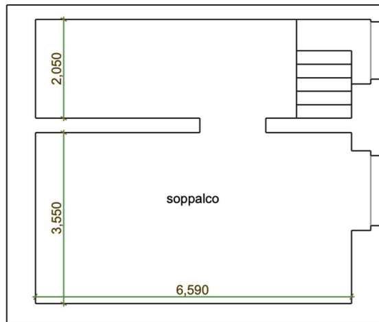
PIANTA PIANO SOPPALCATO
