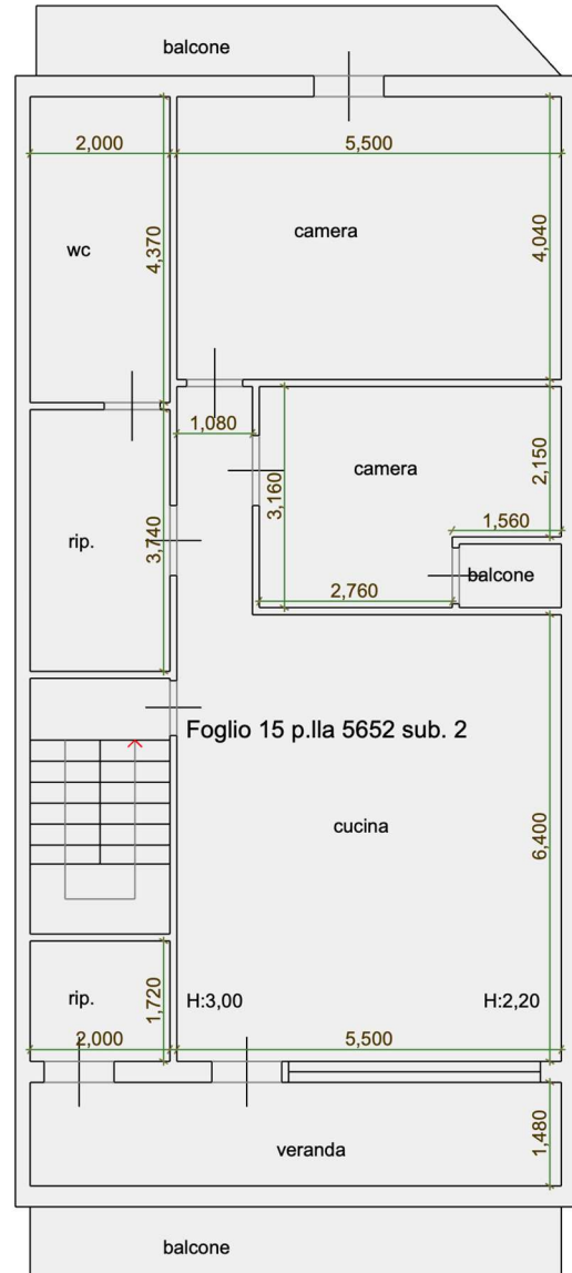
PIANTA PIANO SOTTOTETTO
