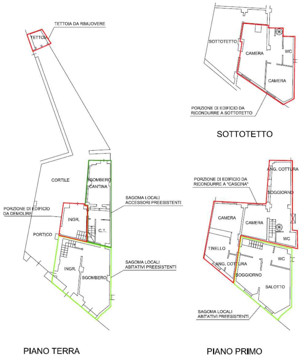
Rilievo di massima stato dei luoghi – porzioni da ripristinare/demolire
