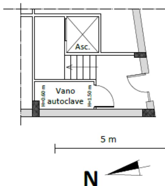
Figura 5 - Planimetria dello stato reale dei luoghi – Vano autoclave Piano Terra
