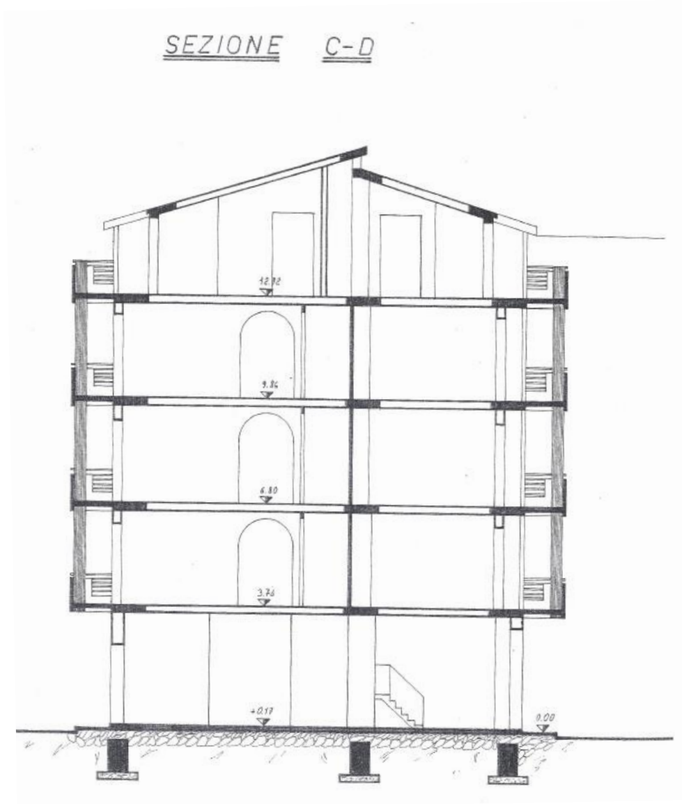
Figura 11 - Sezione trasversale Conc. Ed. n. 33/1995
