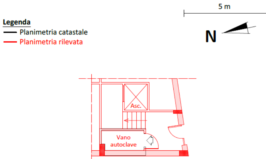
Figura 8 - Sovrapposizione planimetria dello stato reale dei luoghi con la planimetria catastale - Vano autoclave Piano Terra
