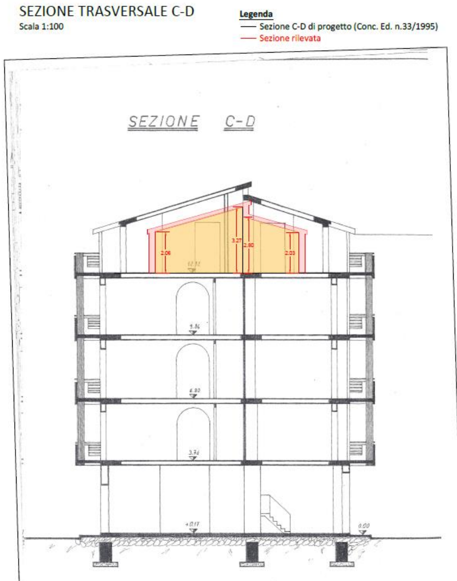
Figura 13 - Sovrapposizione stato reale dei luoghi e progetto autorizzato – Sezione trasversale C-D
