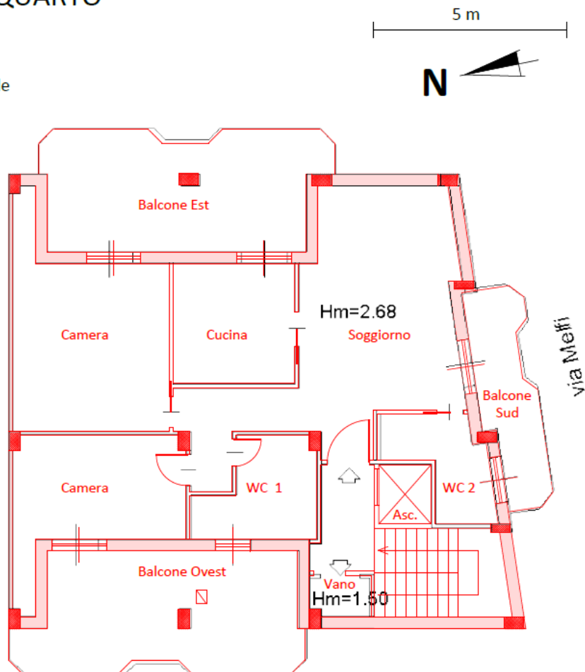
Figura 9 – Sovrapposizione planimetria dello stato reale dei luoghi con la planimetria catastale - Appartamento Piano Quarto
