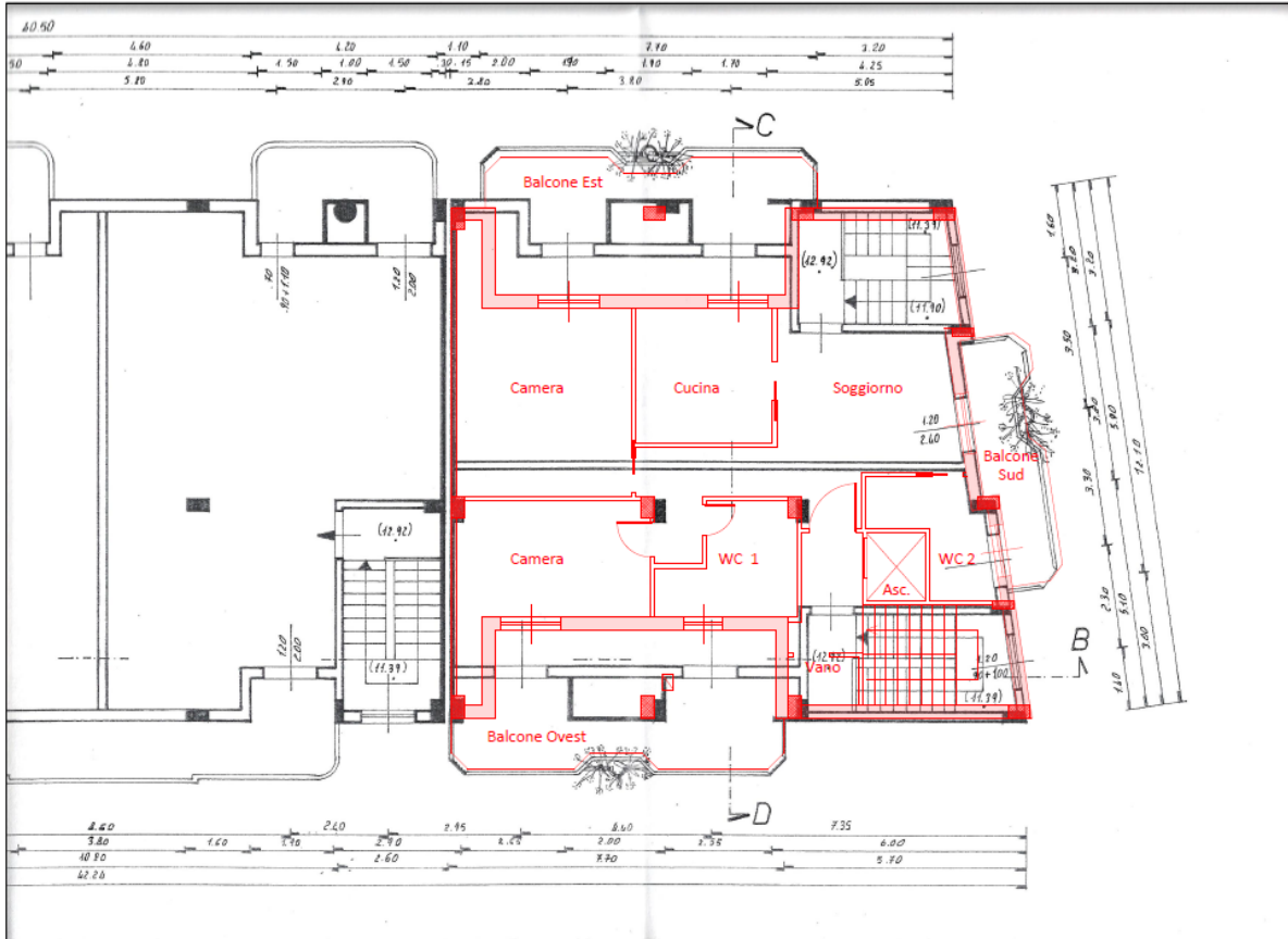
Figura 12 – Sovrapposizione stato reale dei luoghi e progetto autorizzato – Planimetria piano quarto (nota: i lievi disallineamenti rispetto ai fili fissi dei pilastri sono dovuti a distorsioni grafiche degli elaborati di progetto acquisiti presso il Comune)
