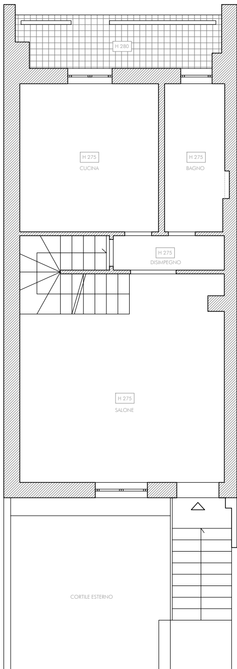
PIANTA PIANO TERRA
