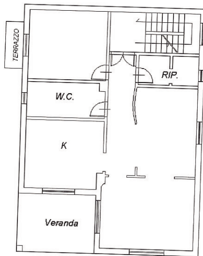
PIANTA PIANO PRIMO H=2,85 m
