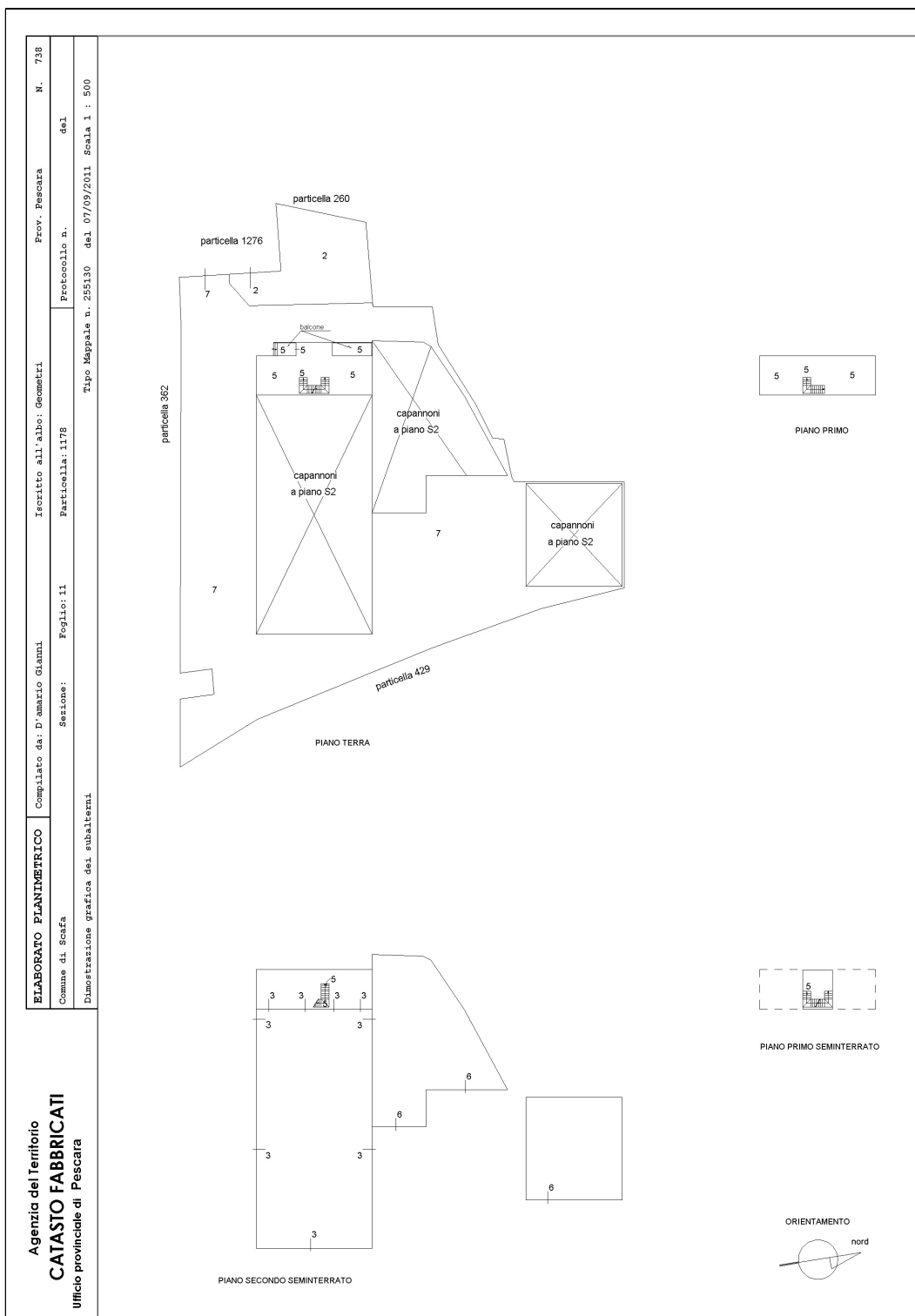
Elaborato Planimetrico – complesso artigianale – Fg. 11 P.Ila 1178 Sub. 2-3-5-6-7
