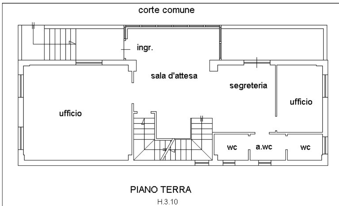
Planimetria catastale - UFFICIO Piano Terra Fg. 11 – P.Ila 1178 – Sub. 5
