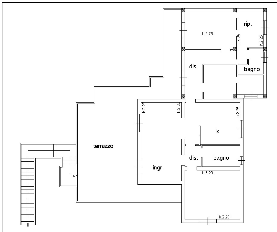
Planimetria catastale – Appartamento piano 1°/sottotetto Fig. 11 – P.IIa 436 Sub 7
