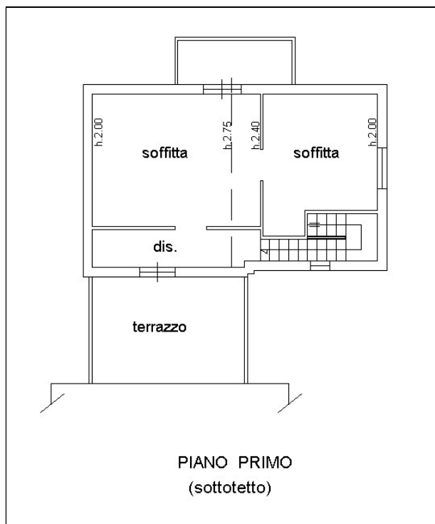
Planimetria catastale – Piano Primo Fig. 11 – P.IIa 924 – Sub. 5
