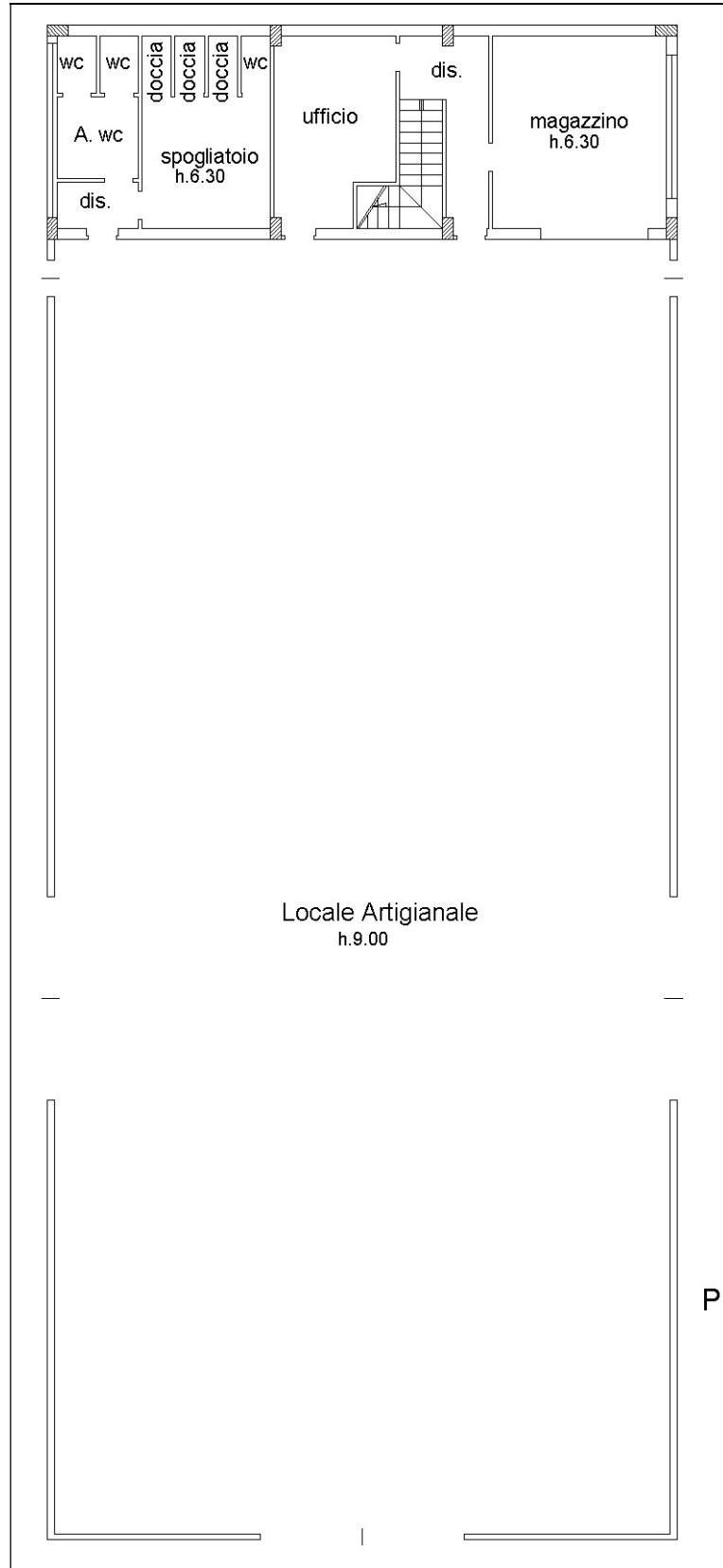
Planimetria catastale - OPificio Piano 2° seminterrato Fig. 11 – P.Ila 1178 – Sub. 3
