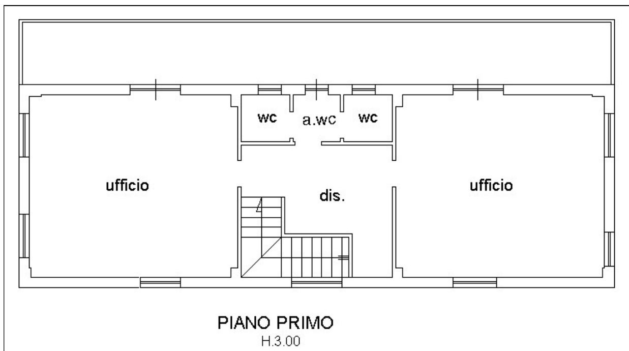
Planimetria catastale - UFFICIO Piano Primo Fg. 11 - P.IIa 1178 - Sub. 5
