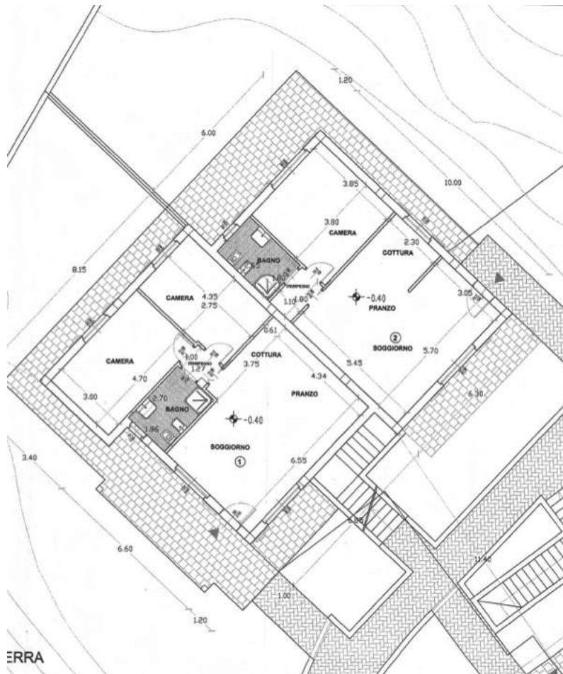
PdC N. 6/2008 NUOVO COMPLESSO RESIDENZIALE - CORPO A: PIANTA PIANO TERRA
