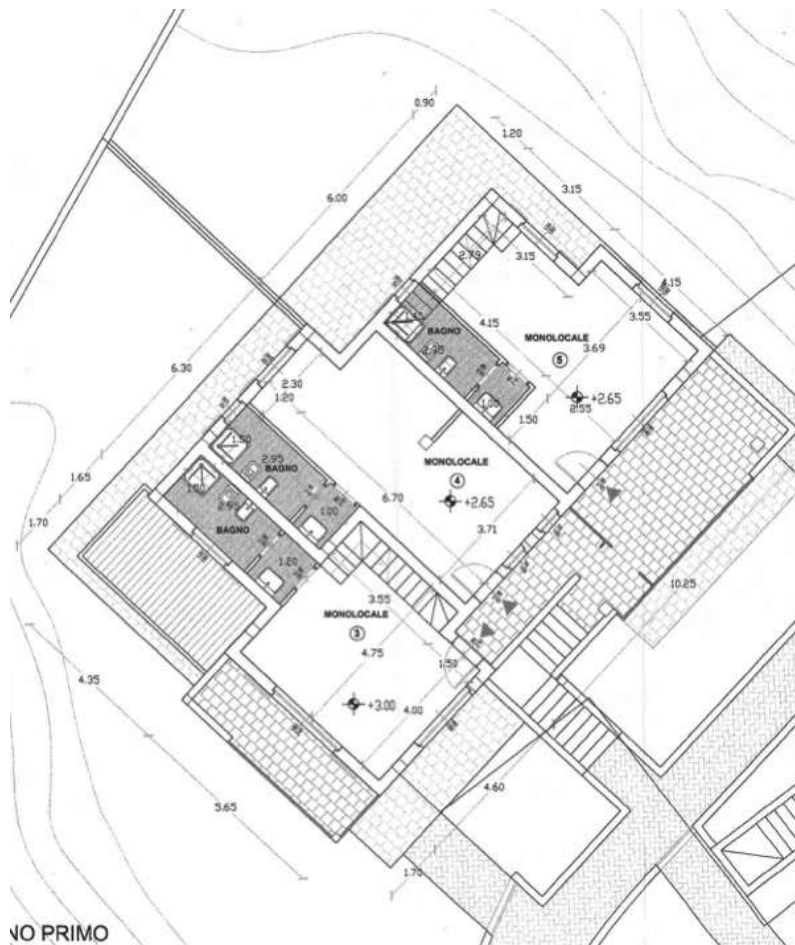
PdC N. 6/2008 NUOVO COMPLESSO RESIDENZIALE - CORPO A: PIANTA PIANO PRIMO
