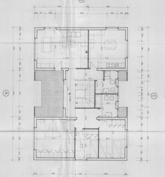
Pianta P. Primo - scala 1:100
