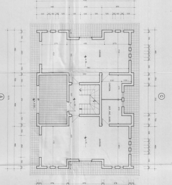
Pianta P. Terra - scala 1:100
