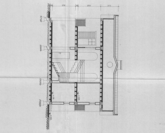
Sezione Tronca - scala 1:100
