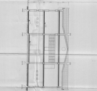
Sezione Lunga - scala 1:100
