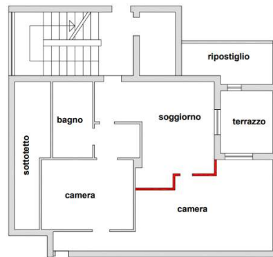
Elab. 6 – Evidenza dei tramezzi demoliti
