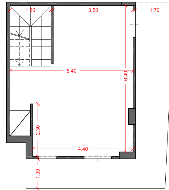
PIANTA PIANO PRIMO H= 2.82m
