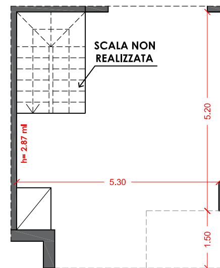
PIANTA PIANO SOTTOTETTO Hm= 2.23 m
