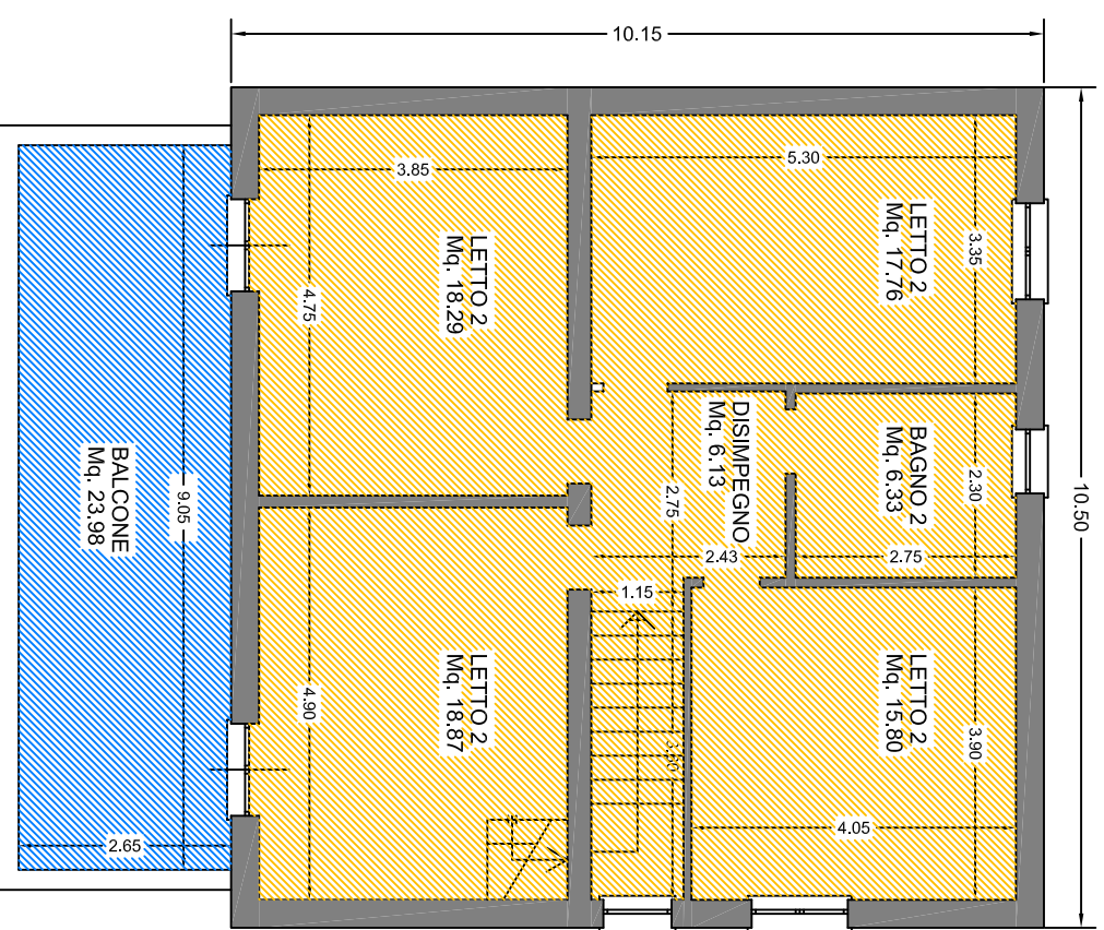
Pianta piano primo quota +120 cm _rilievo del 15.07.2022 N.B. il bagno è stato realizzato in assenza di titolo abilitativo
