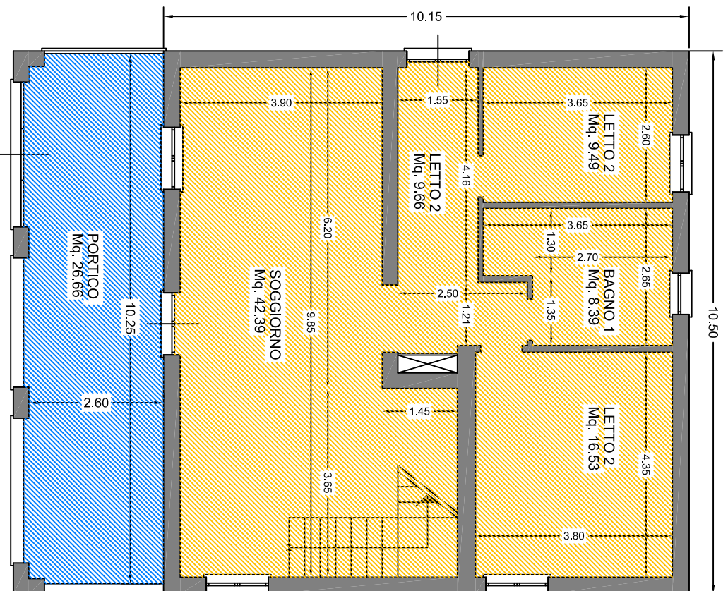
Pianta piano terra _rilievo del 15.07.2022
